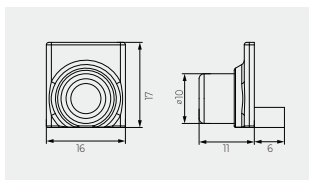
Integral End Cap (IP67)
